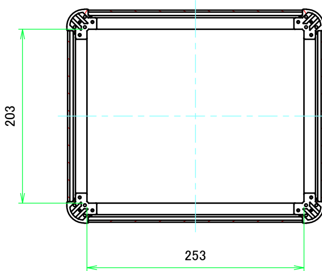
C-C ( 1:4.5 )
